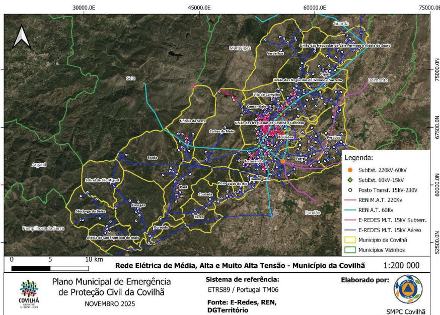
Figura 36 – Rede Elétrica do Município da Covilhã
