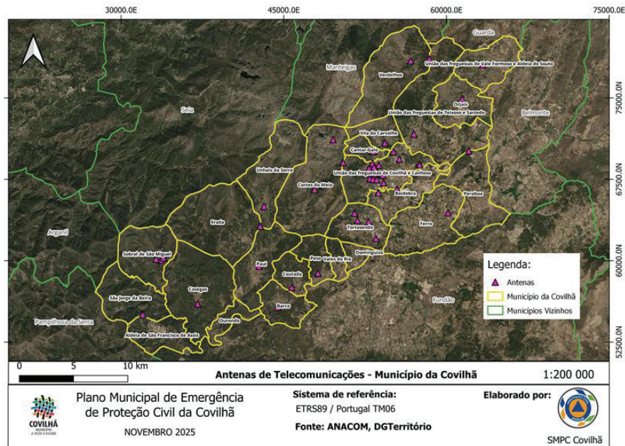
Figura 64 – Antenas de telecomunicações – Município da Covilhã
